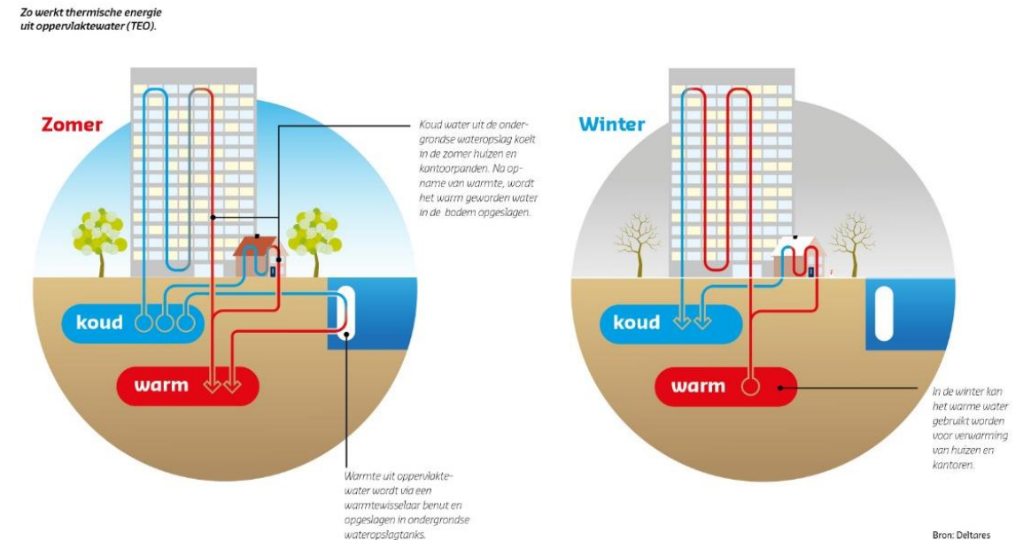
Figuur 2: Schematische weergave van TEO met een WKO in de winter en in de zomer. Bron: Ontwerphandleiding Aquathermie TEO - WarmingUP (2022)
